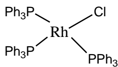
Figura 1. Complejo de organorodio propuesto como catalizador hipotético en reacción de hidrogenación de propileno.
